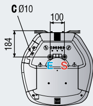
Vista inferior
